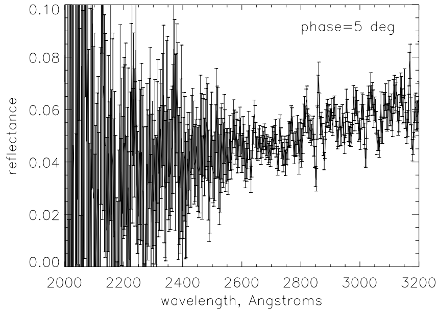
Juno IUE LWR05679LL
