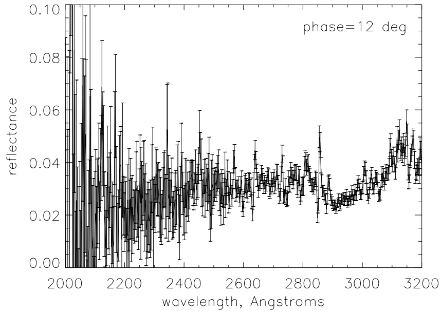
Juno IUE LWR06487LL
