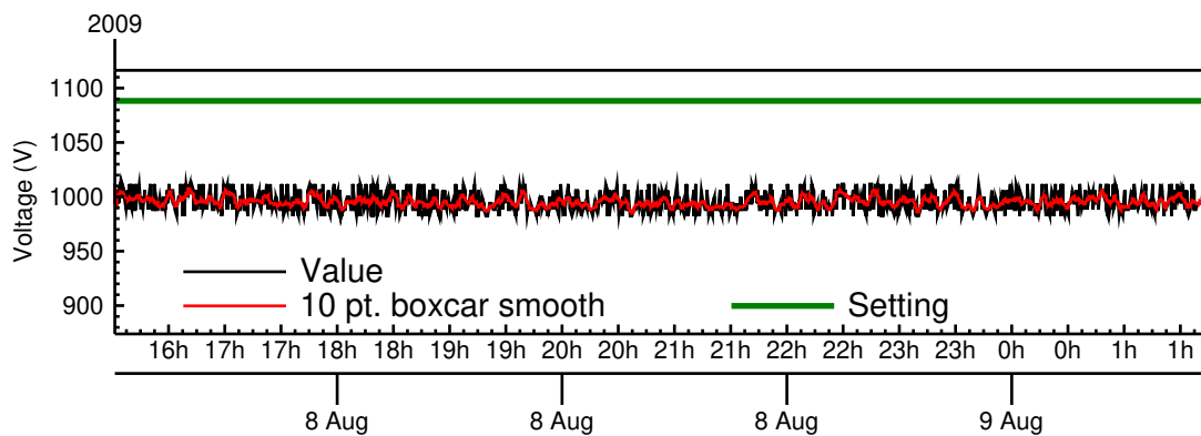
HVPS1 (+Z)
