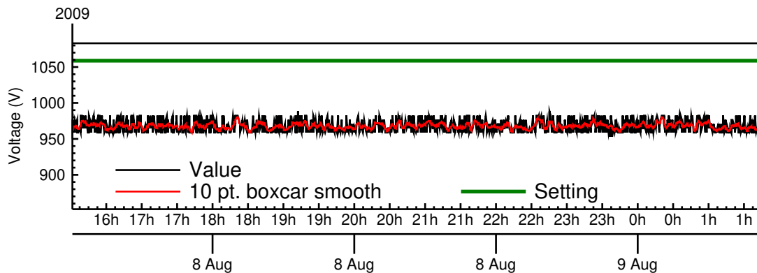
HVPS4 (-Z)
