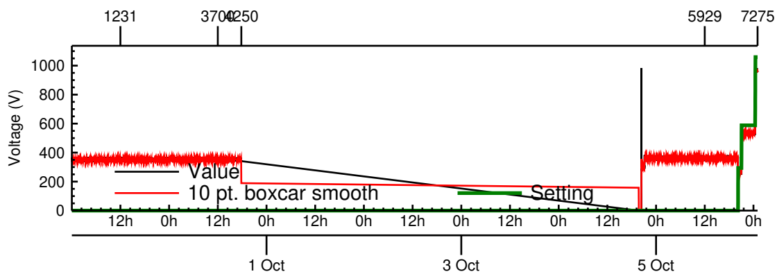
HVPS4 (-Z)
