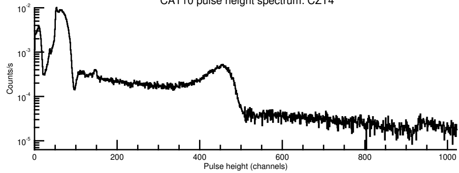
CAT10 pulse height spectrum: CZT4
