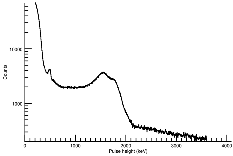
CAT10 CZT composite
