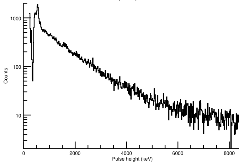
BGO-CZT pair spectrum: BGO
