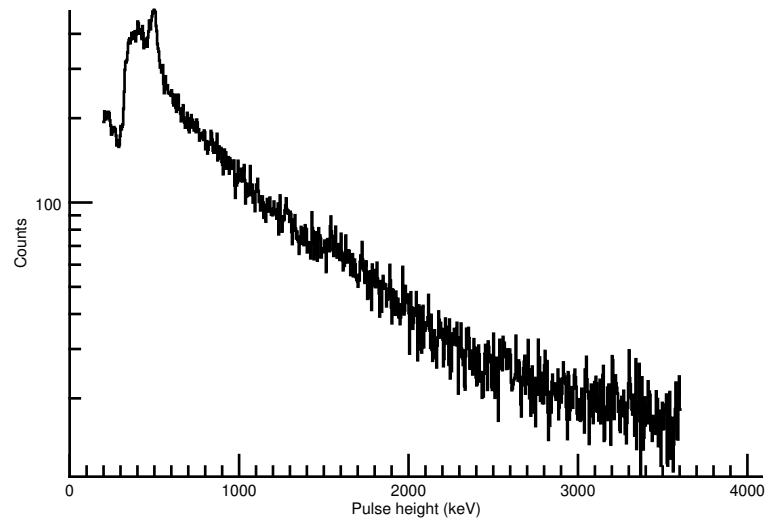
BGO-CZT pair spectrum: CZT
