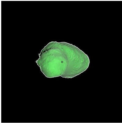
Figure 437: ST_2423386961_v.fits
