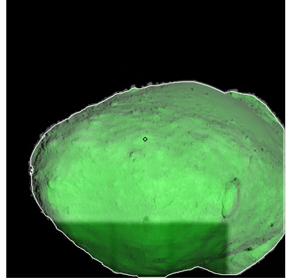
Figure 588: ST_2495287635_v.fits
