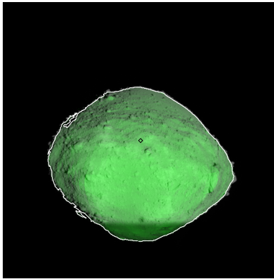
Figure 599: ST_2506502552_v.fits
