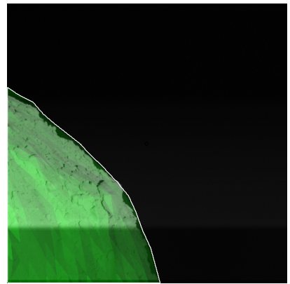
Figure 618: ST_2539489658_v.fits
