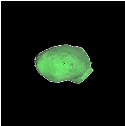
Figure 347: ST_2421281610_v.fits
