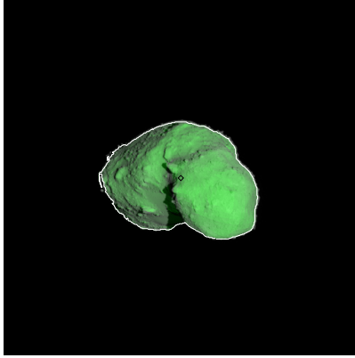
Figure 281: ST_2420740941_v.fits
