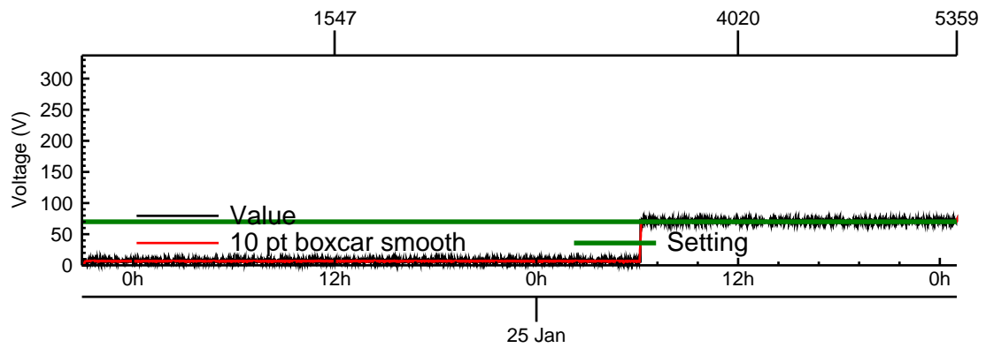
HVPS70 (CZT grid bias)
