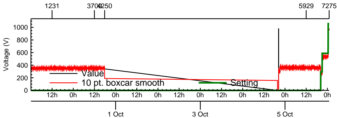
HVPS4 (-Z)
