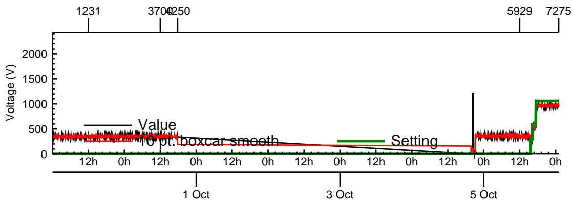
HVPS1 (+Z)
