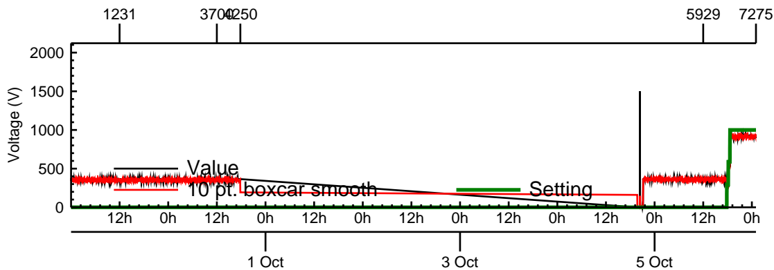
HVPS2 (-Y)
