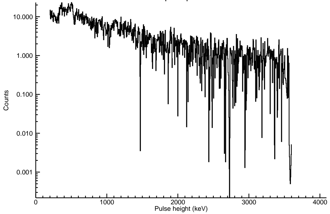
BGO-CZT pair spectrum: CZT
