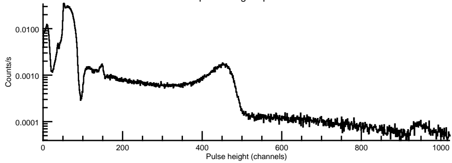
CAT10 pulse height spectrum: CZT4
