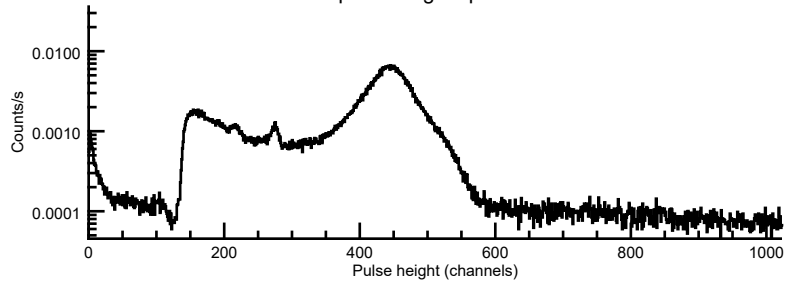
CAT10 pulse height spectrum: CZT6
