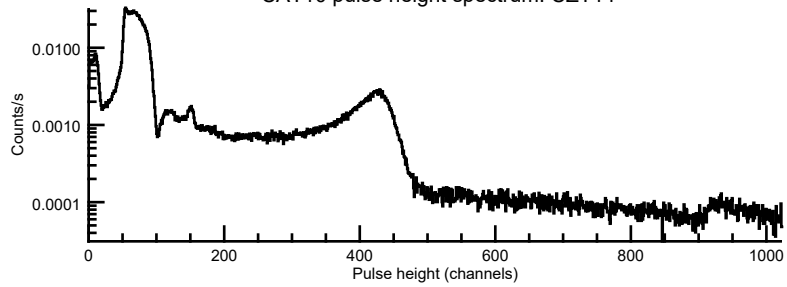
CAT10 pulse height spectrum: CZT4
