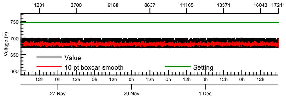
HVPS5 (BGO)
