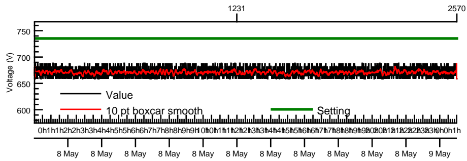
HVPS5 (BGO)
