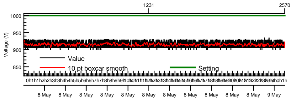
HVPS6 (CZT)
