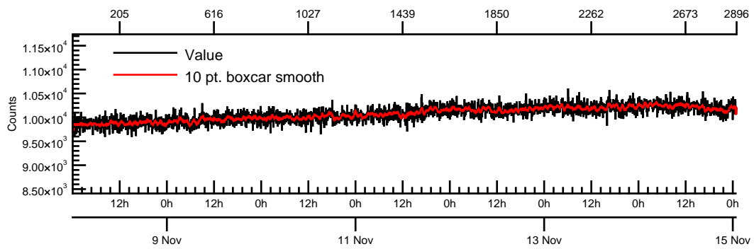
Valid CZT events (CAT10)
